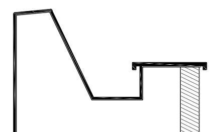
VERDECKTE ÜBERLAUF - RINNE MIT BEIDSEITIGER AUFKANTUNG INFINITY / WASSERFALL
