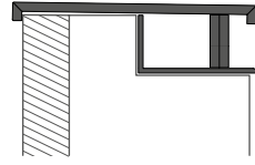
Schwimmbadkopf Verdeckte Überlaufrinne Bordo piscina
