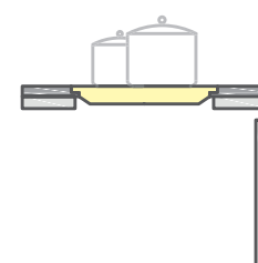
HO. Kochfeld flächenbündig HO. Piano cottura a filo
